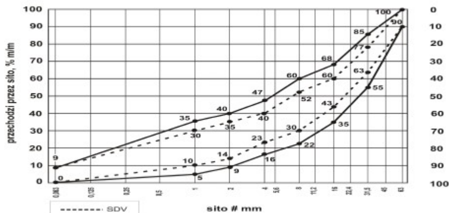
Rys. 3. Mieszanka niezwiązana 0/63 do warstw podbudowy zasadniczej
