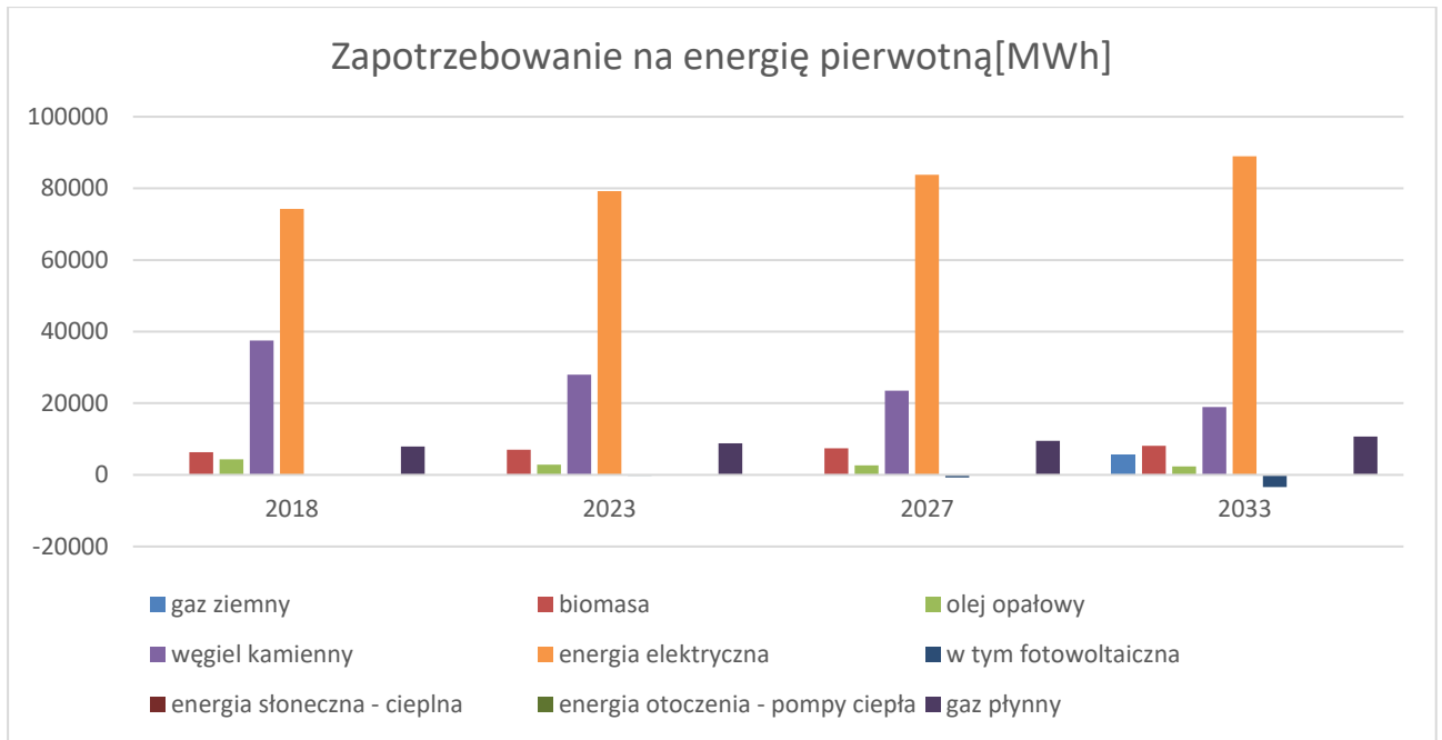
Rys. 30 Zapotrzebowanie na energię pierwotną - perspektywy
