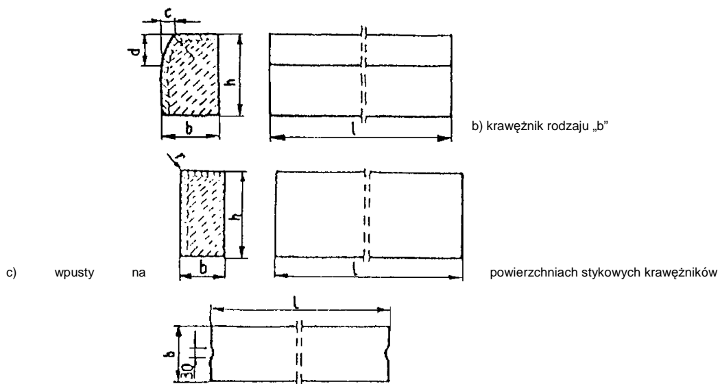
Rys. 1. Wymiarowanie krawężników
